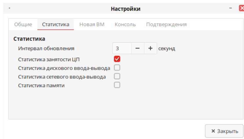
Рисунок 10.24 – Вкладка Статистика
