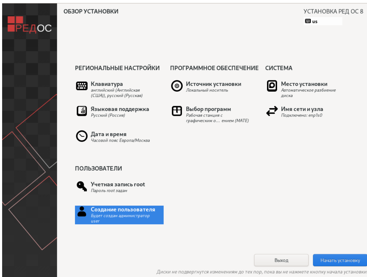
Рисунок 4.13 — Конфигурация ОС
