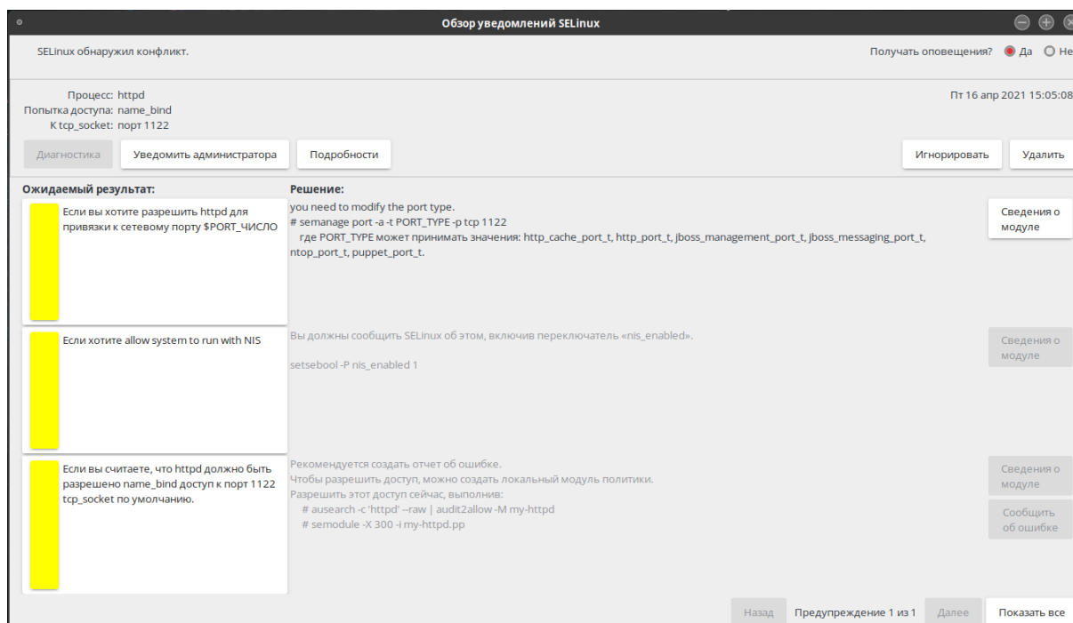
Рисунок 6.3 — Окно уведомлений
