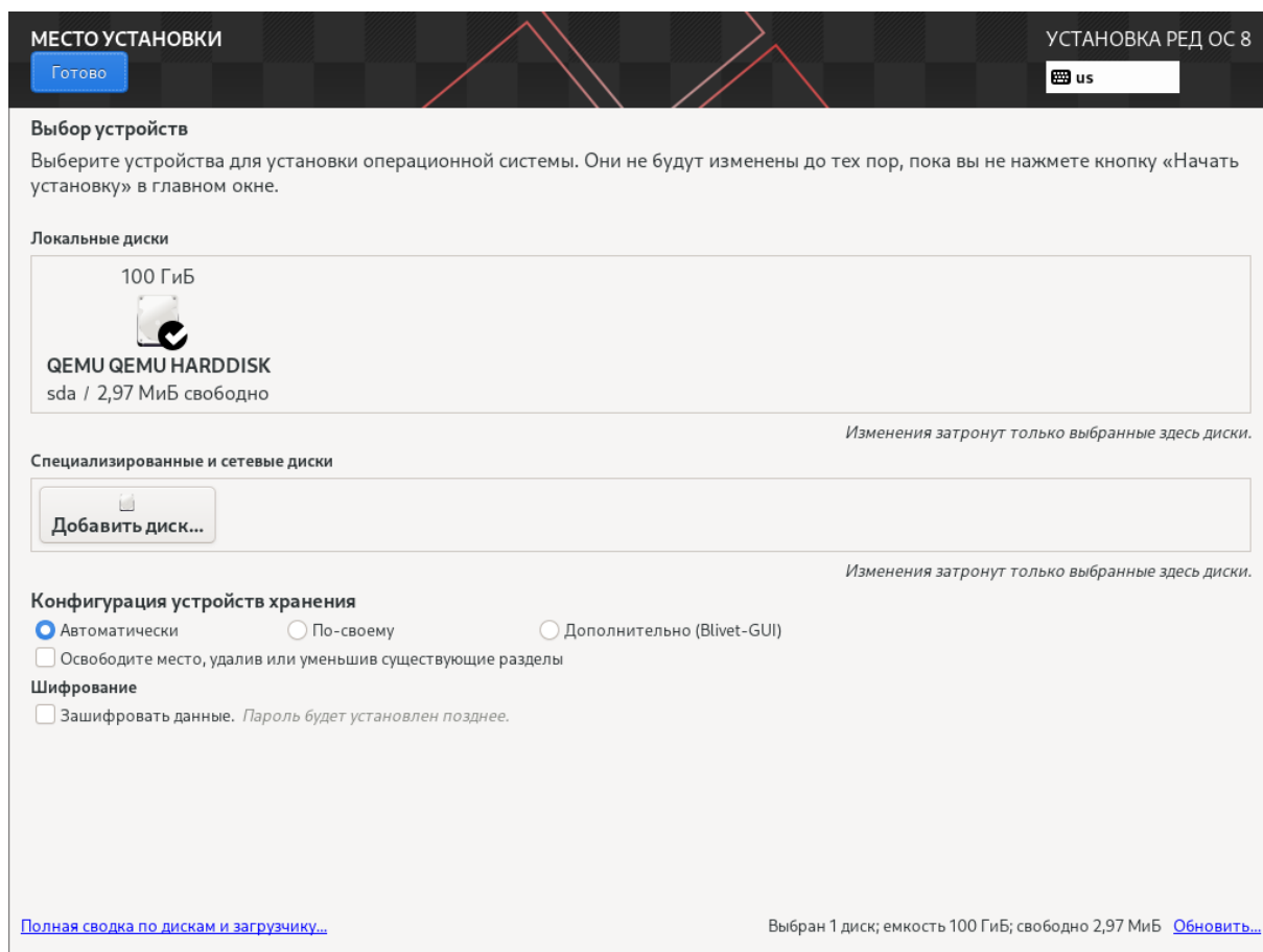
Рисунок 4.9 — Расположение установки
