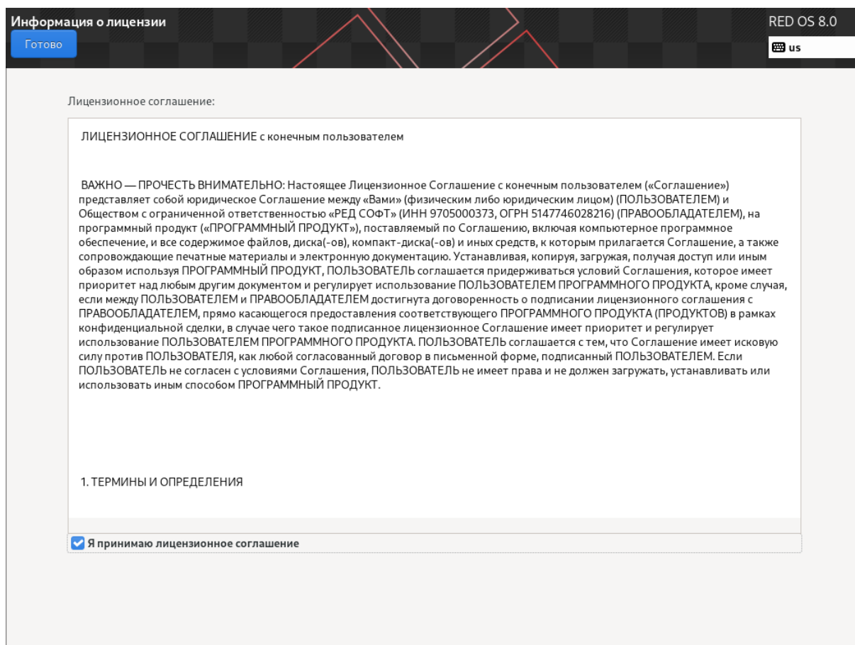
Рисунок 4.15 — Лицензия
