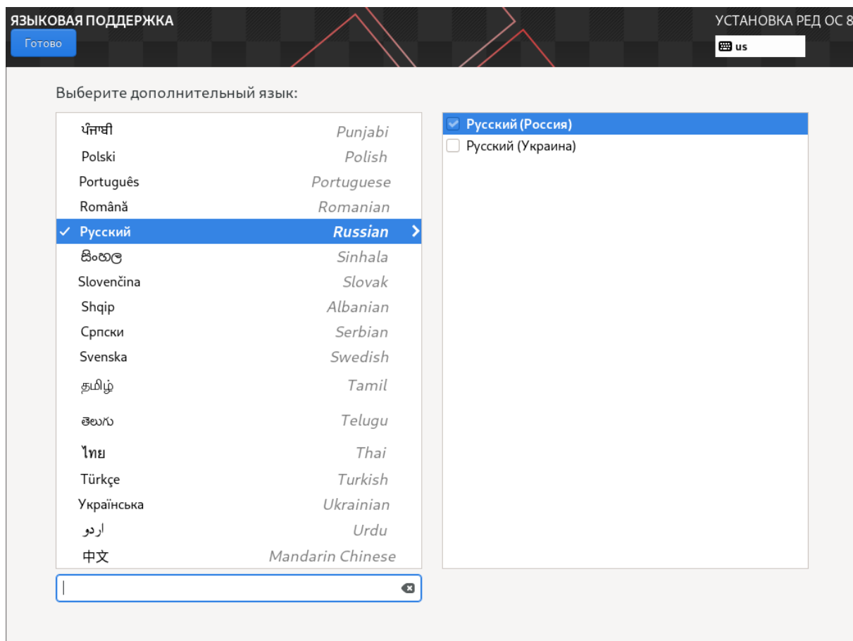
Рисунок 4.6 — Языковая поддержка
