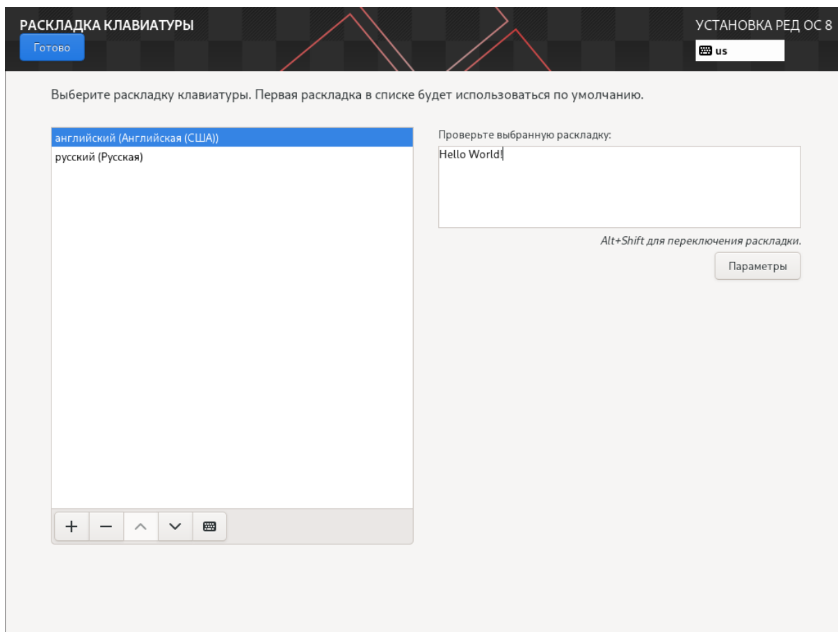
Рисунок 4.5 — Раскладка клавиатуры
