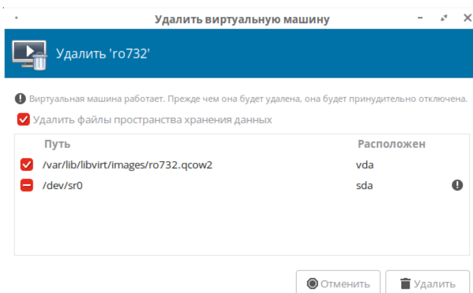
Рисунок 10.39 – Удаление VM
