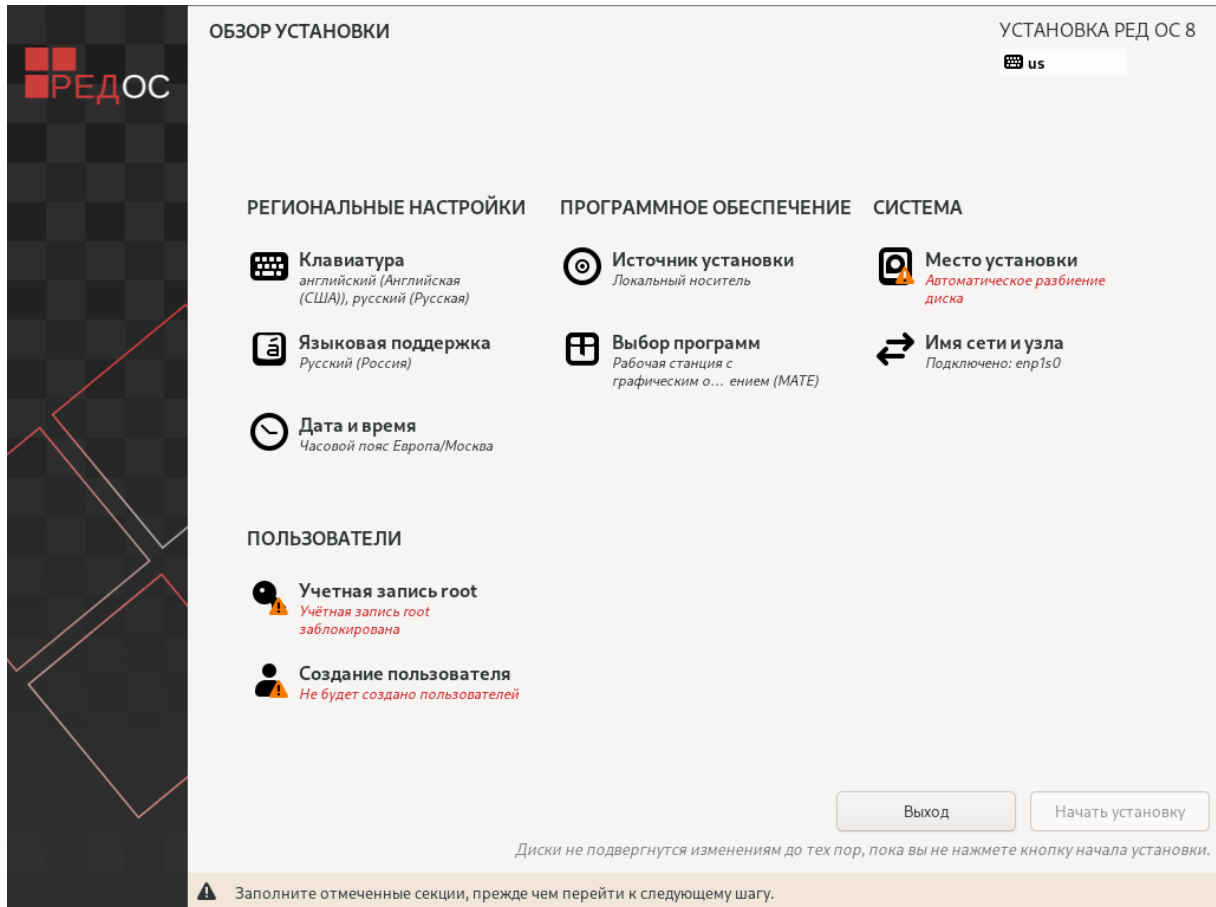
Рисунок 4.3 — Обзор установки
