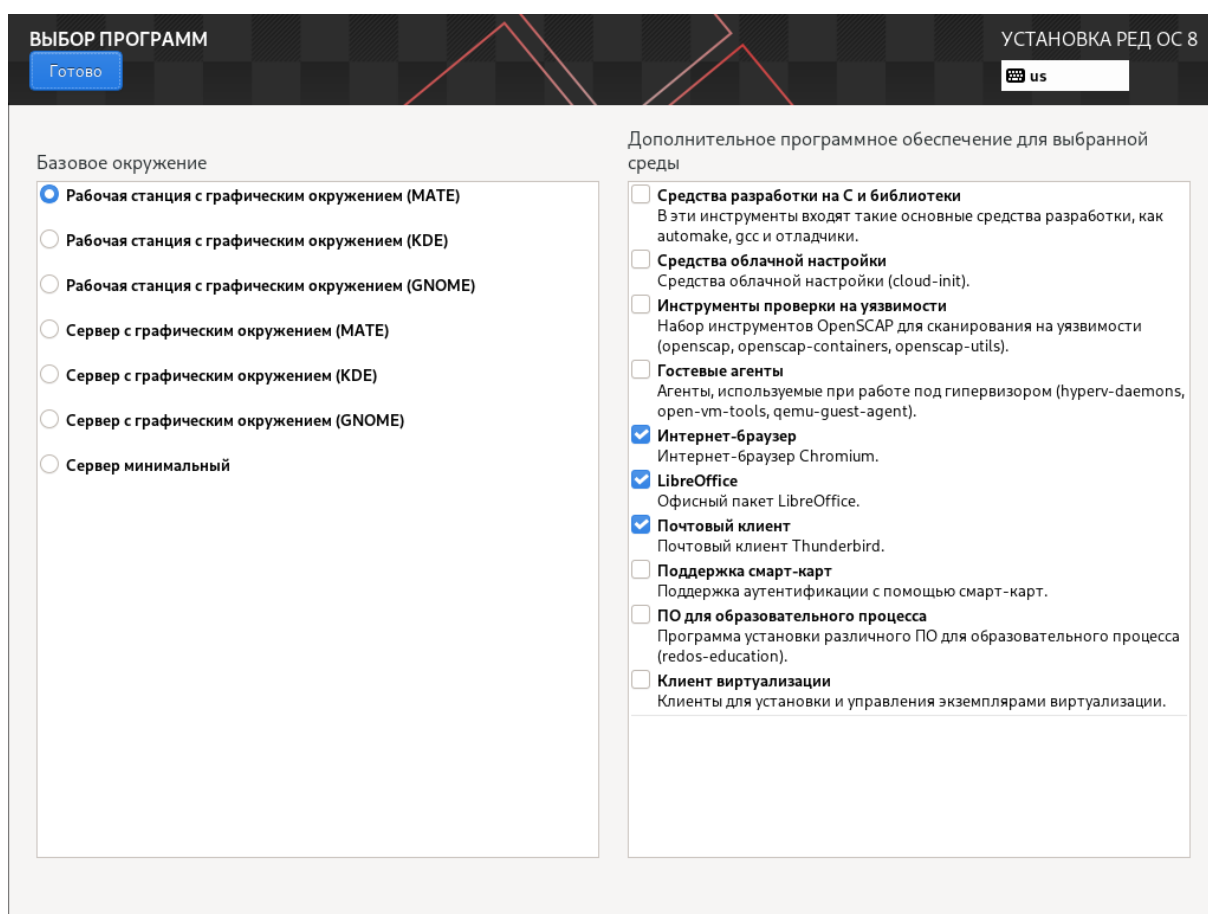
Рисунок 4.8 — Выбор программ
