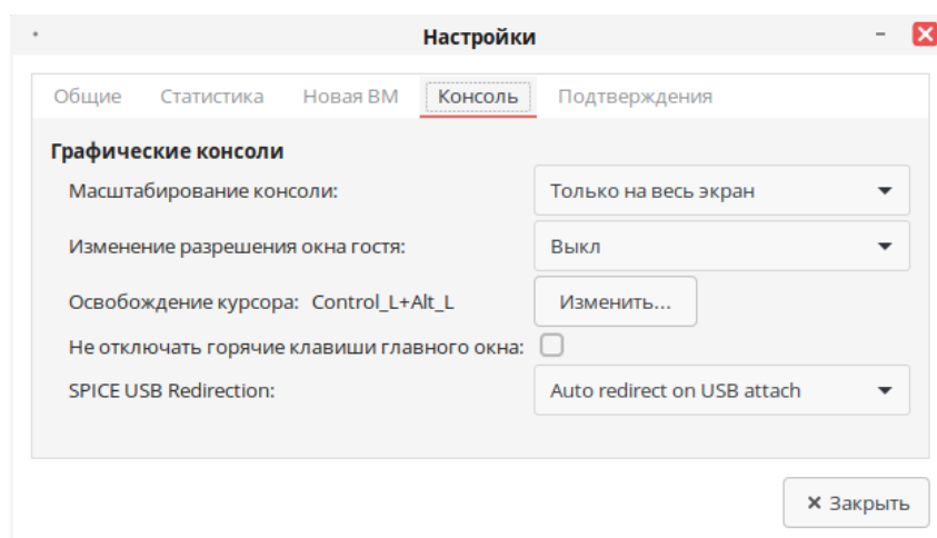
Рисунок 10.26 – Вкладка Консоль
