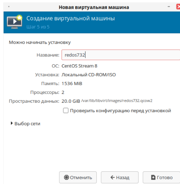
Рисунок 10.13 – Проверка параметров
